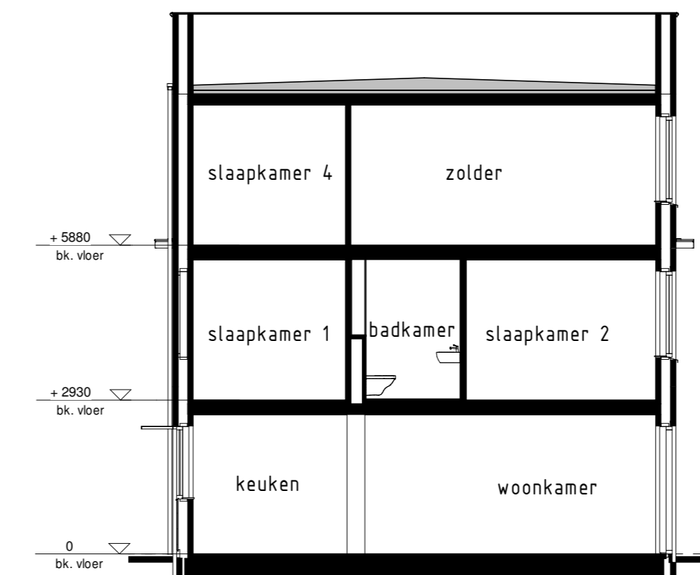
DOORSNEDE 10C - 10C 1:100
