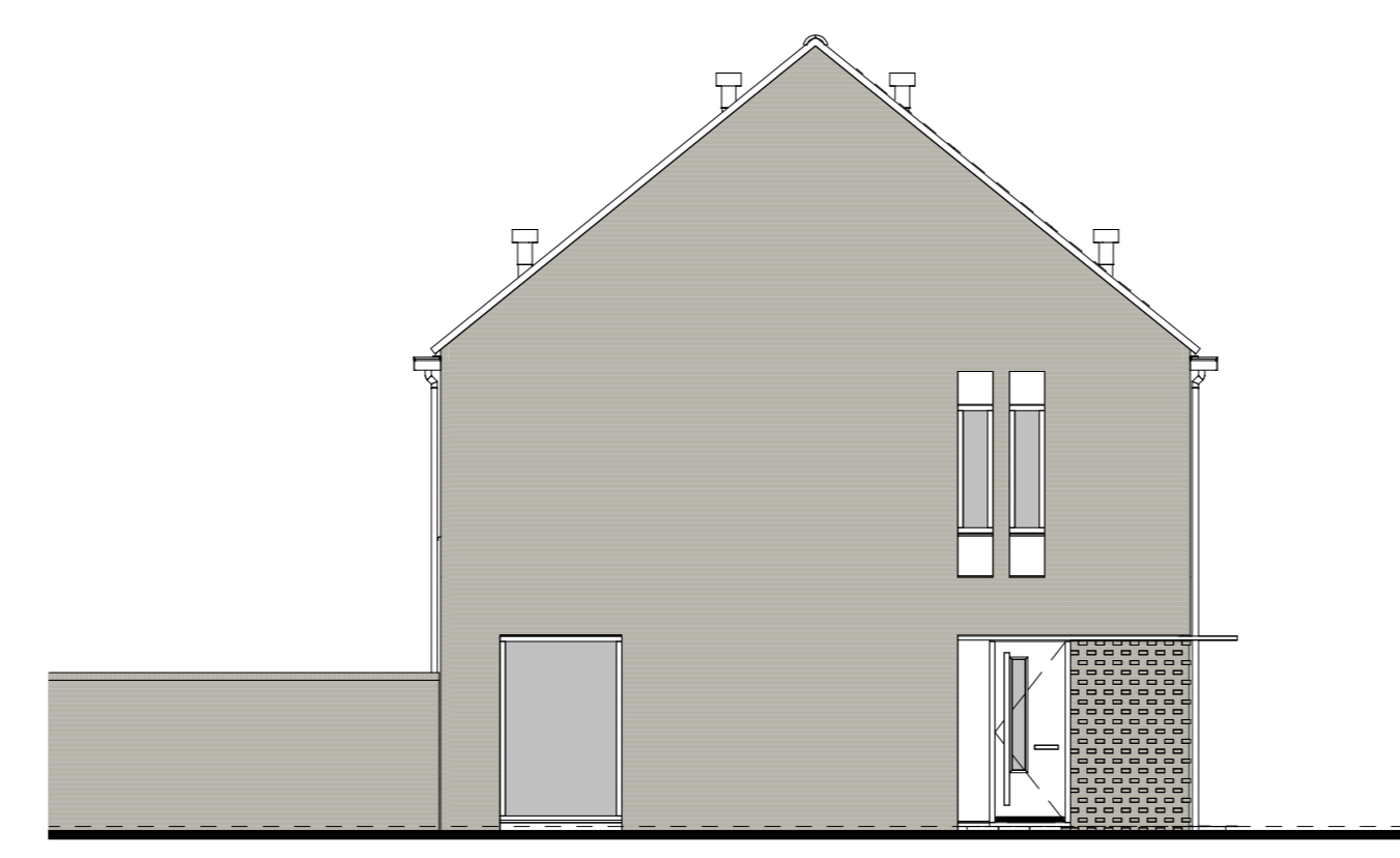
LINKERGEVEL 1:100
