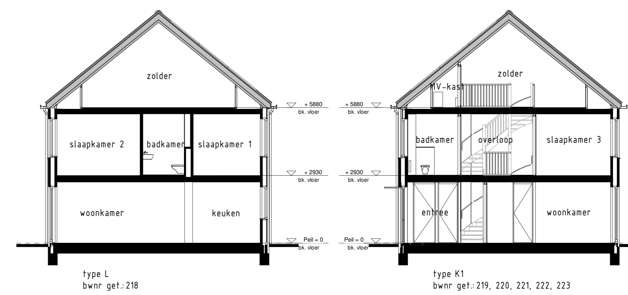
DOORSNEDE 10A - 10A 1:100
