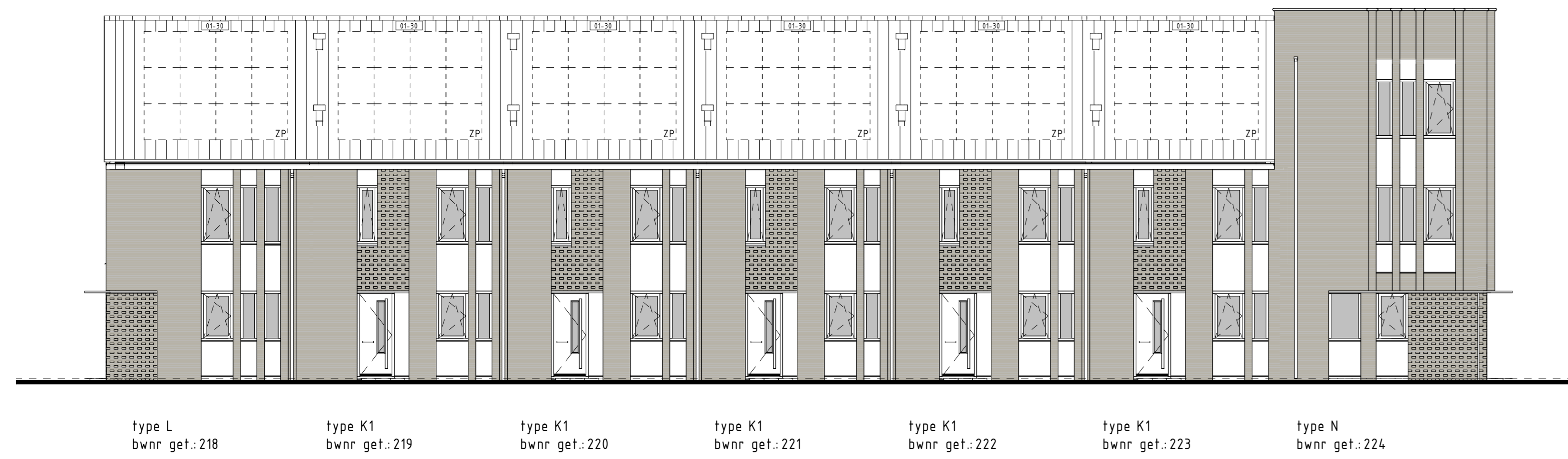
VOORGEVEL 1:100
