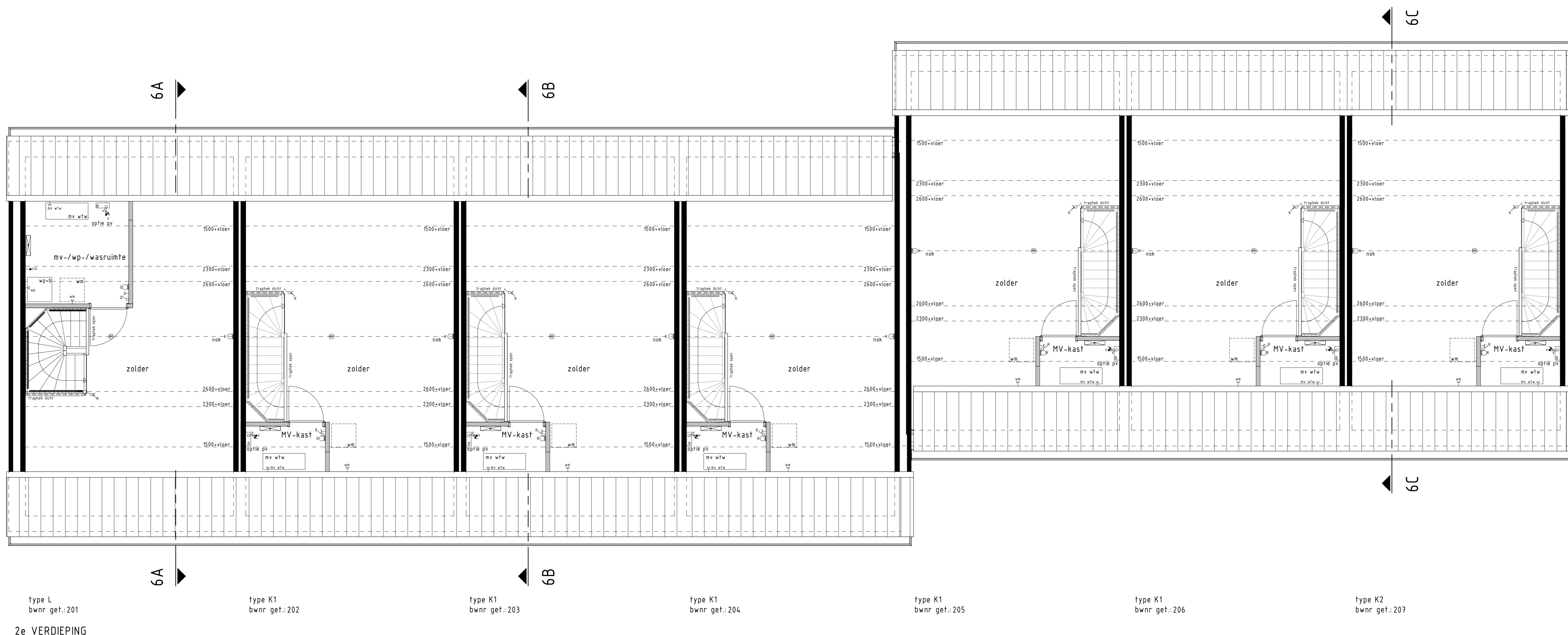
2e VERDIEPING
